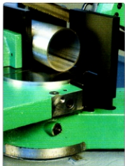
Spannstock mit Schnellannäherung mit einstellbarer Leiste
