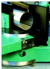
(*) Spannstockschultern können nach hinten verstellt werden so dass die max. Schnittkapazität (340 x 180 mm) erreicht wird. Eingekerbte Mass-Skala mit einfacher Ablesung
